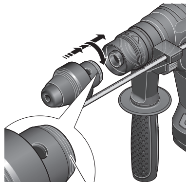
識別溝 (2本または3本)
